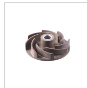
EG-P187 Φ107 H30 8 blades
